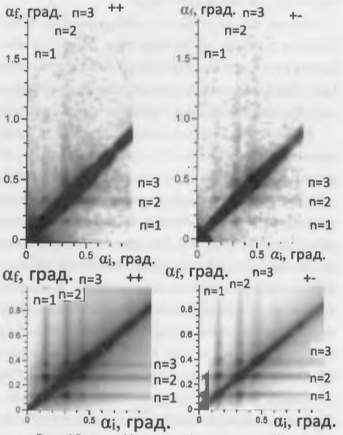
Рис. 18. Интенсивность нейтронов, отражённых от магнитного волновода в поле 1 Э. Левая колонка - мода "++", правая колонка - мода "+-". Верхняя строка - эксперимент, нижняя строка - расчёт.
