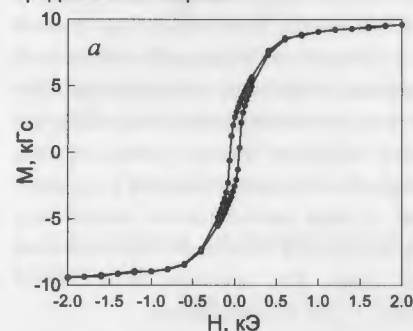
Рис. 8. Характеризация плёнки \text{Ru}(500 \text{ нм}) : а) данные VSM; б) коэффициенты отражения нейтронов "+" (тёмные точки) и "-" (светлые точки) в магнитном поле 20 Э; в) коэффициенты отражения нейтронов в магнитном поле 4.4 кЭ.
