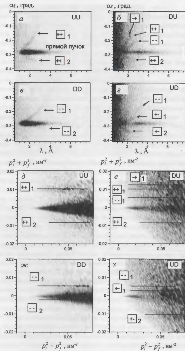
Рис. 3. Экспериментальные данные преломления нейтронного пучка в плёнке FeAlSi: а-г) инструментальные координаты; ж-з) квадратичные нормированные координаты. UU, DD, UD и DU обозначают режим спин-флипперов вкл. (U) и выкл. (D). Индексы 1 и 2 соответствуют разным границам раздела.
