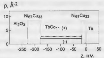
Рис. 19. ПДР нейтронов для волноводной структуры с ферромагнитной плёнкой TbCo 11 (150 нм).
