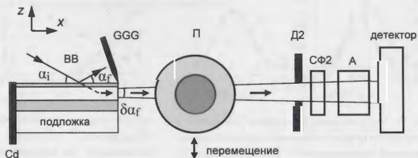
Рис. 25. Схема экспериментальной установки по сканированию магнитной проволоочки микропучком: Cd – кадмиевая пластина; BB – волновод; GGG – кристалл галлий-гадолиний-гранат; П – проволоочка; Д2 – вторая диафрагма; СФ2 – второй спин-флиппер; А – анализатор.
