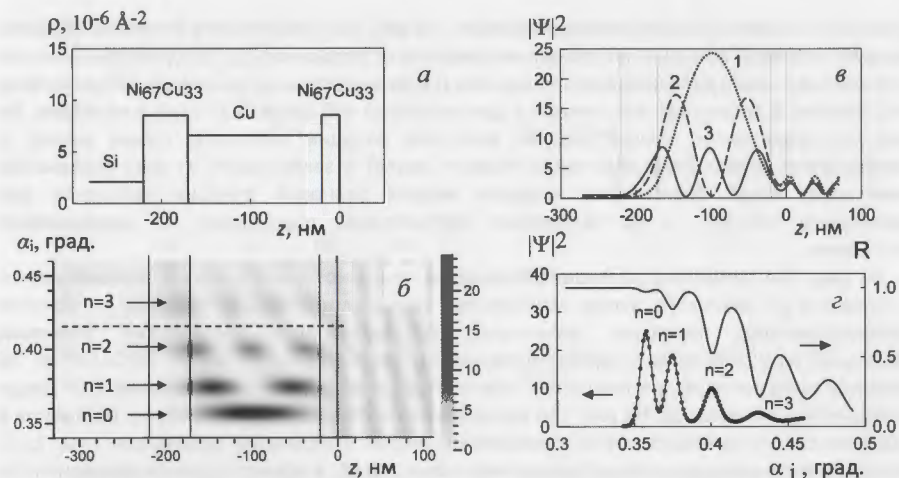
Рис. 12. Расчёты для волновода Ni 67 Cu 33 (20 нм)/Cu(150)/Ni 67 Cu 33 (50)/Si(подложка). а) ПДР. б) Квадрат модуля волновой функции нейтронов. в) Квадрат модуля волновой функции нейтронов для резонансов n=0 (кривая 1), n=1 (кривая 2) и n=2 (кривая 3) в зависимости от координаты z. з) Квадрат модуля волновой функции нейтронов (левая шкала) и коэффициент отражения (правая шкала) в зависимости от угла скольжения начального пучка.
