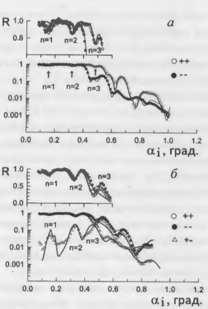
Рис. 17. Коэффициенты отражения поляризованных нейтронов от магнитного волновода Py(20 нм)/Ti(80)/Py(50)//glass для длины волны 4.52 Å во внешнем магнитном поле: (а) 100 Э; (б) 1 Э.
