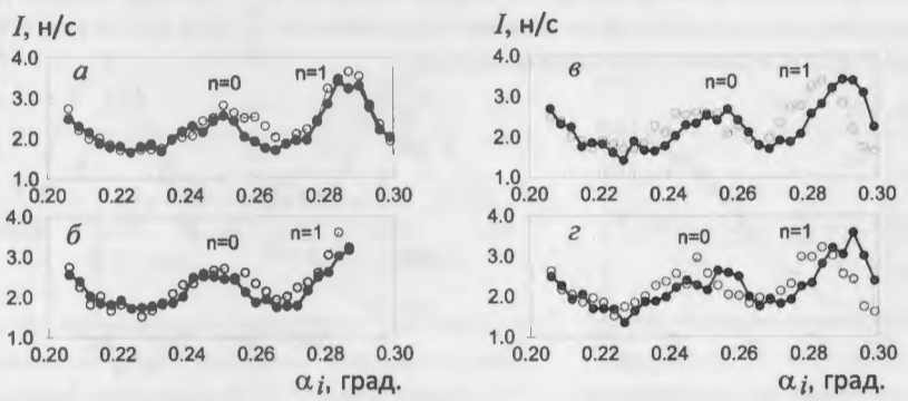
Рис. 20. Интенсивность микропучков "+" (тёмные символы) и "- " (светлые символы) как функция угла скольжения начального пучка во внешнем магнитном поле: а) 451 Э; б) 530 Э; в) 620 Э; г) 640 Э. Ошибка равна размеру символов. Длина волны нейтронов 4.26 Å. Волновод Ta(3 нм)/Ni 67 Cu 33 (15)/TbCo 11 (150)/Ni 67 Cu 33 (50)//Al 2 O 3 (подложка).
