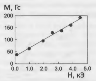
Рис. 24. Намагниченность плёнки TbCo 5 (150 нм), полученная в эксперименте на рефлектометре поляризованных нейтронов NREX.
