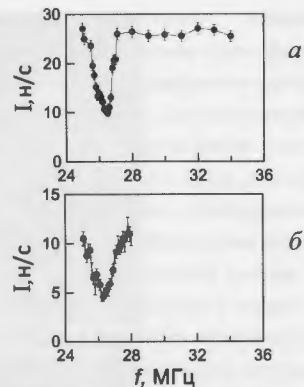
Рис. 7. Интенсивность нейтронов в максимуме пика зеркально отражённого пучка в зависимости от частоты приложенного внешнего магнитного поля: а) спин "+"; б) спин "-".
