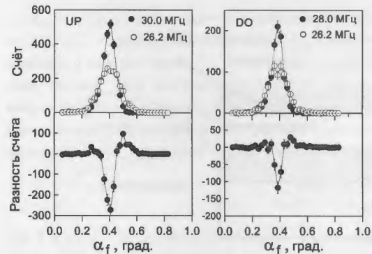
Рис. 9. Счёт отражённых нейтронов при резонансной частоте (светлые точки) и вне резонанса (тёмные точки) и их разность.
