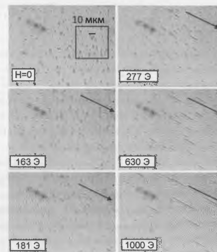
Рис. 4. Фотография поверхности плёнки Gd/Fe//\text{стекло} (подложка) с магнитным коллоидом в технике Биттера. Стрелкой показано направление приложенного внешнего магнитного поля.
