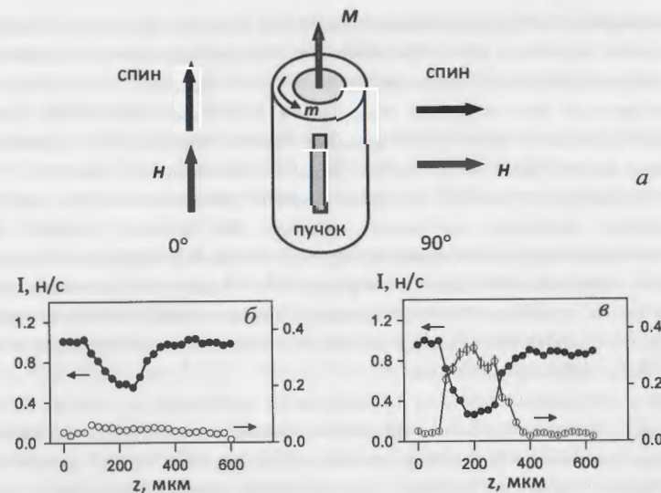
Рис. 26. Пространственное сканирование магнитной проволоочки поляризованным микропучком нейтронов. а) Геометрия эксперимента с магнитной проволоочкой. б) Интенсивность микропучка нейтронов во внешнем поле, параллельном оси проволоочки. в) Интенсивность нейтронов во внешнем поле, перпендикулярном оси проволоочки. Тёмные точки и левая шкала соответствуют спиновому переходу "++", а светлые точки и правая шкала соответствуют спиновому переходу "-+".
