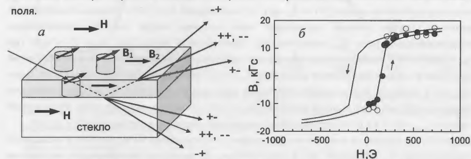
Рис. 5. Плёнка Gd/Fe//\text{стекло} (подложка). а) Геометрия эксперимента. б) Магнитная индукция в кластерах в зависимости от внешнего магнитного поля. Линия - данные VSM для всей плёнки, светлые точки - данные из расщепления пучка при отражении, тёмные точки - данные из расщепления пучка при преломлении.
